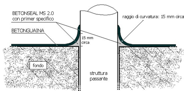
Figura 4 – Trattamento delle strutture passanti
