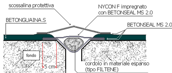
Figura 9 - Realizzazione di giunti di dilatazione strutturali.
