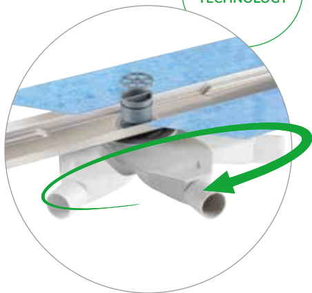
Sifone orientabile a 360° 360° swivelling siphon
